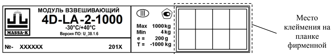
Рис. 15.1 - Планка фирменная
