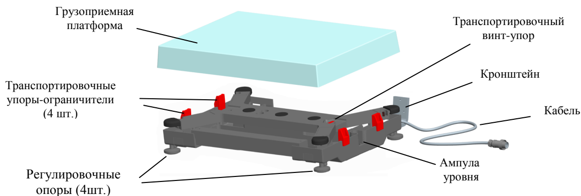
Рис. 3.1 - Модуль взвешивающий
