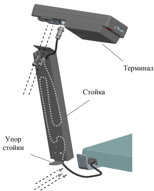
Рис. 3.2 - Сборка весов
